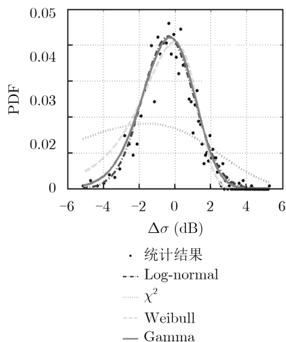
图 7 昆虫RCS起伏幅度PDF拟合
