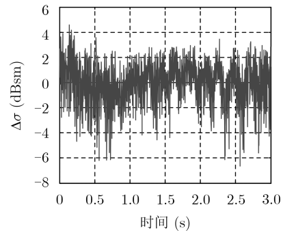
(b) 昆虫RCS起伏幅度
