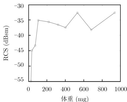
(a) 水平极化RCS
