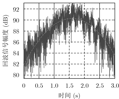
— 回波信号 --- 拟合数据 (a) 昆虫回波信号幅度及拟合值
