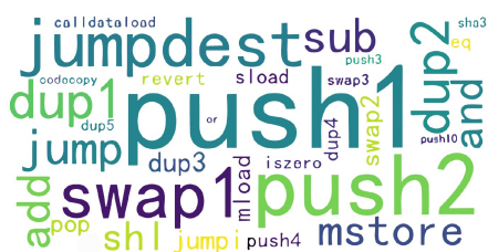
(a) 游戏类别合约操作码1
