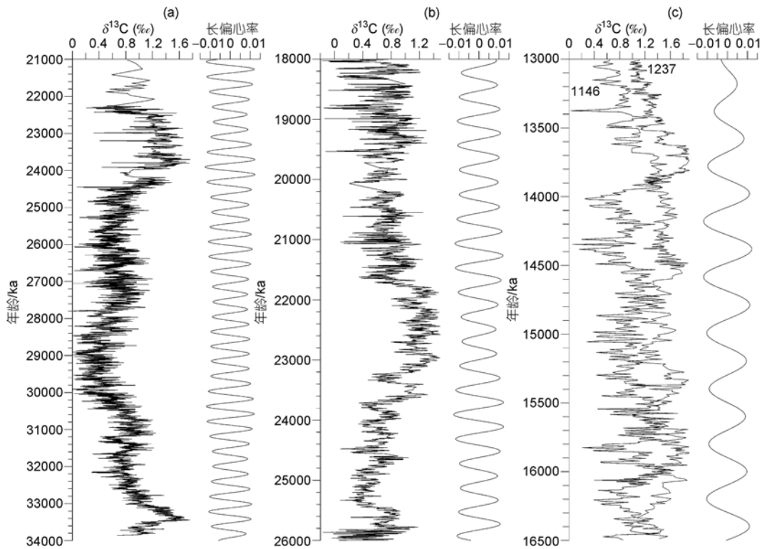
图6 新生代大洋碳同位素的40万年偏心率长周期
