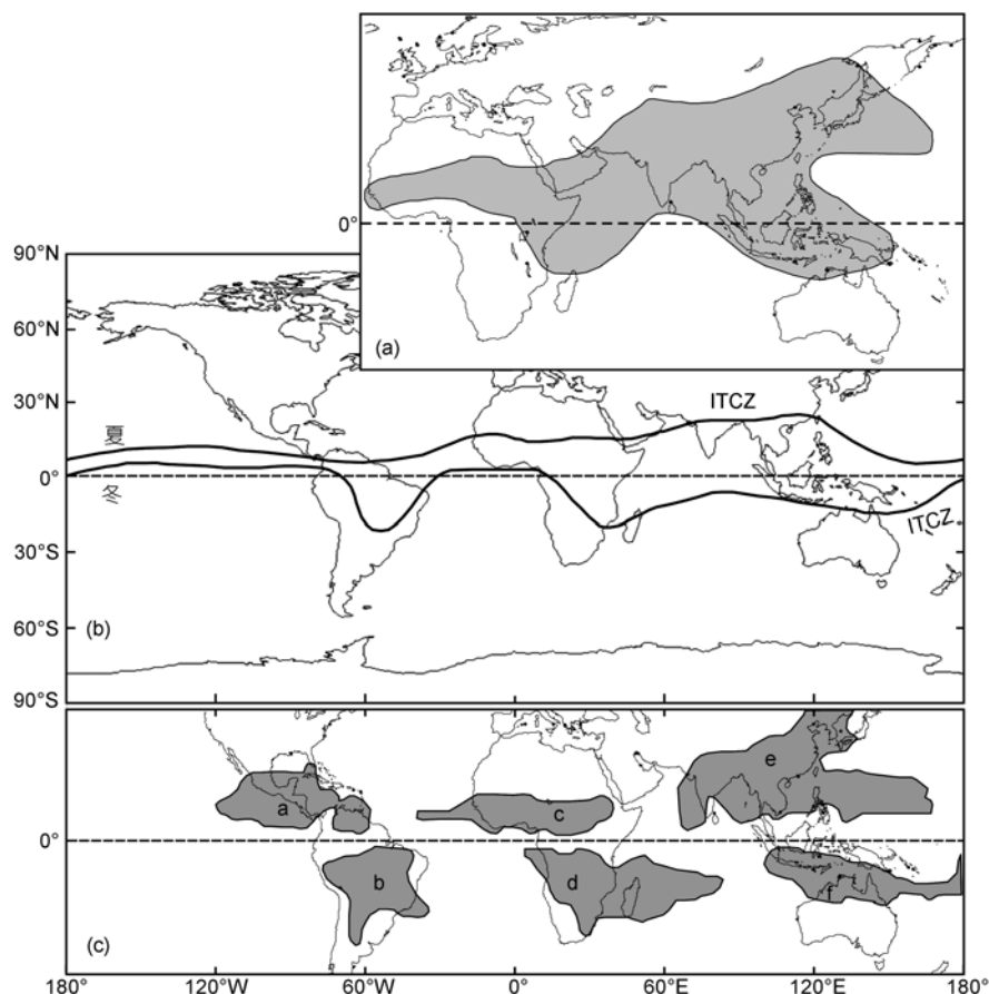
图1 现代的季风系统分布
