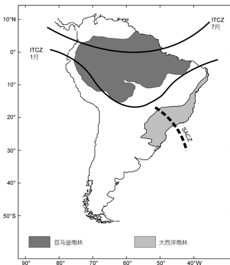
图 2 南美季风与 ITCZ 的关系
