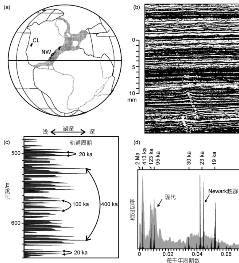
图 10 北美晚三叠世“超级季风”的地质证据
