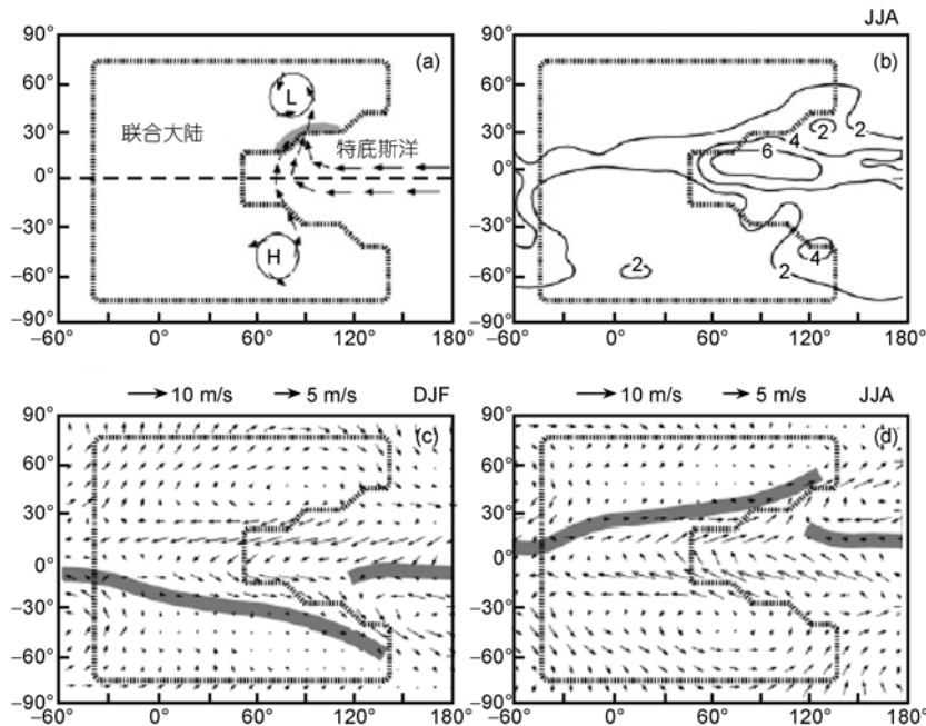
图 9 联合大陆的“超级季风”示意图
