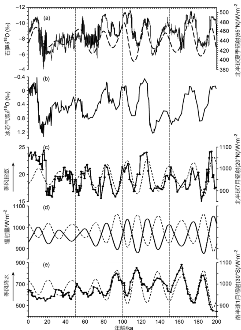
图4 近20万年来南北半球季风的岁差周期
