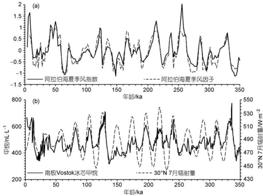
图5 35万年来季风史的不同记录
