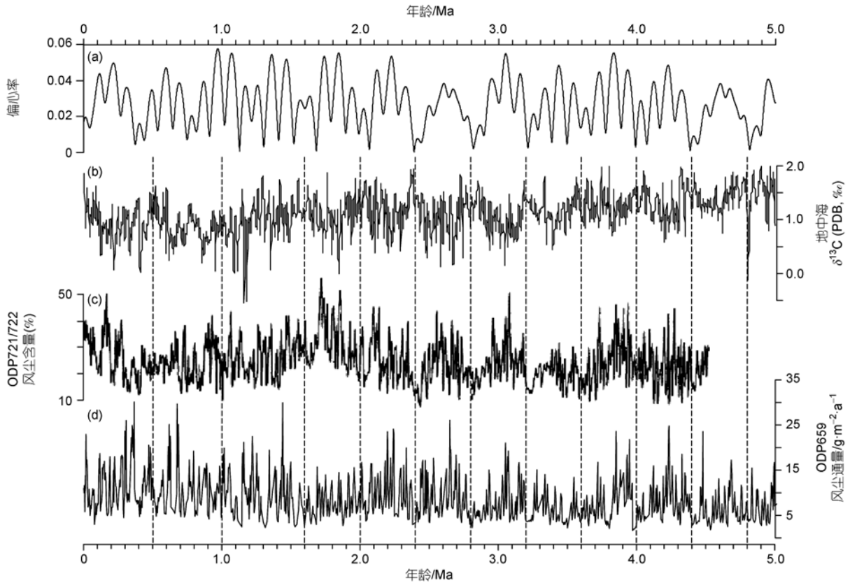
图7 500万年来偏心率长周期与全球季风的关系
