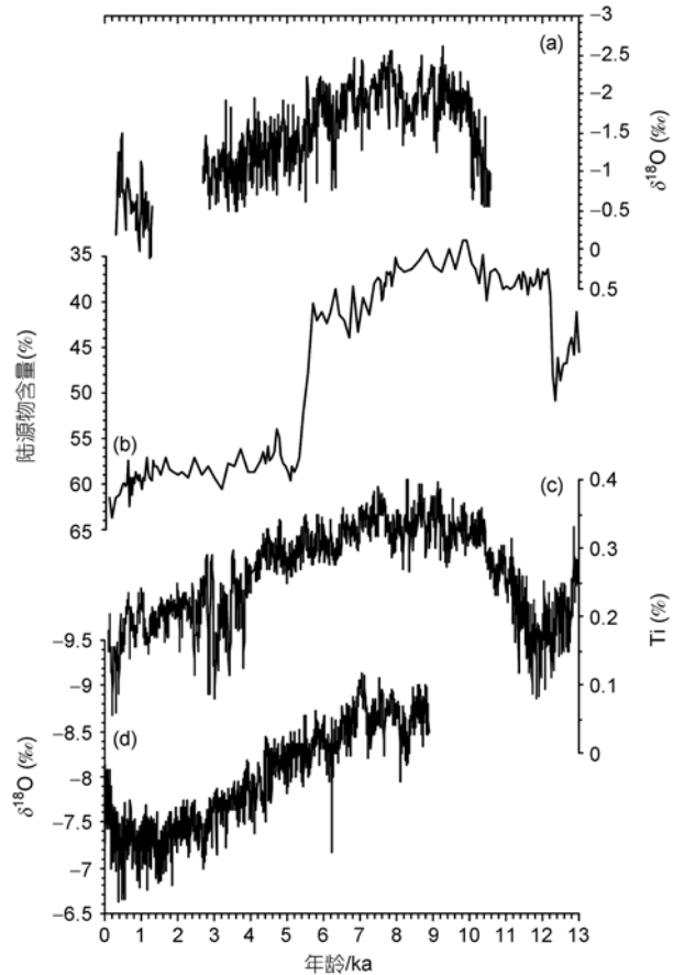
图3 全新世北半球季风演变共同趋势
