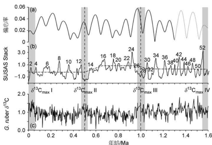
图 8 近 160 万年来大洋碳储库变化的 3 个阶段
