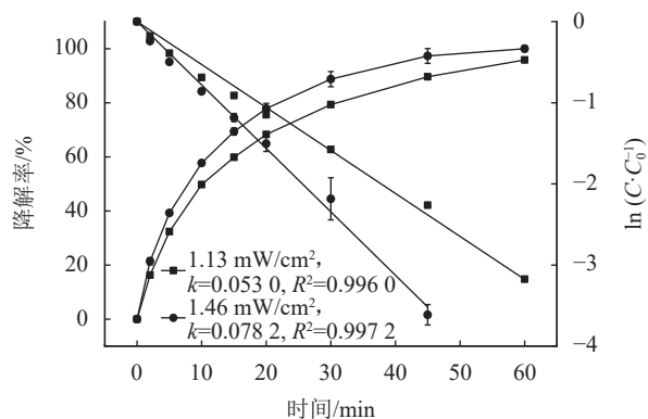
图 5 UV光强对降解SAC的降解率影响
