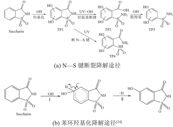
图 3 SAC降解路径及机理推断图
