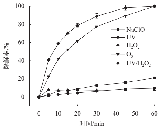
(a) 不同氧化工艺对 SAC 的降解效率
