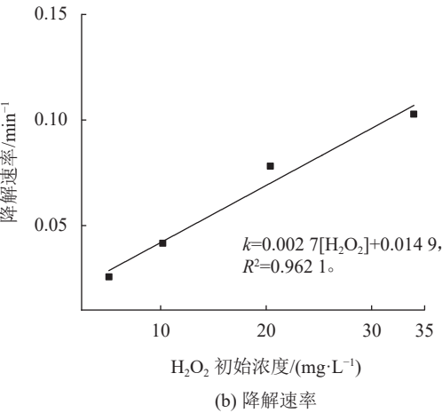
图 4 H 2 O 2 初始浓度对降解SAC的降解率和降解速率的影响
