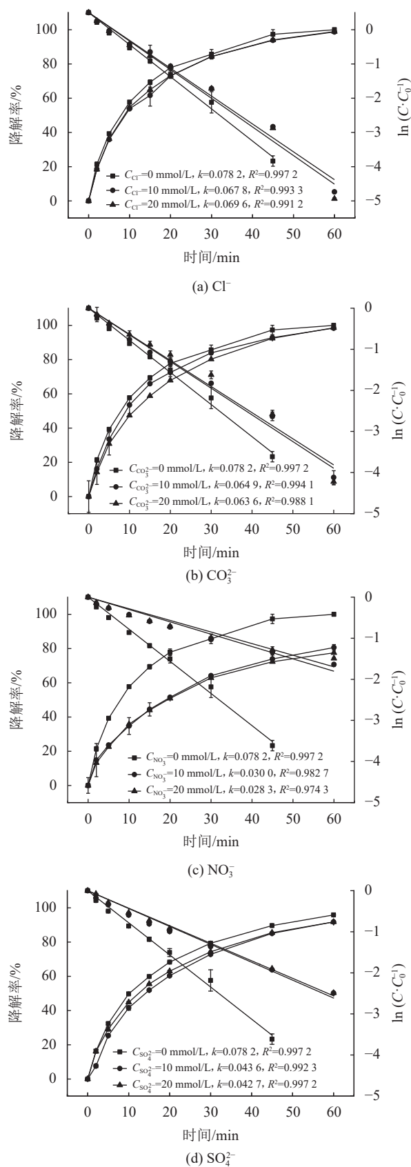
图9 4种阴离子对降解SAC的降解率的影响
