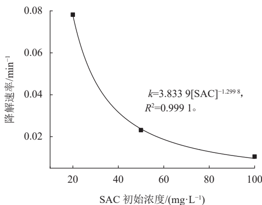
(b) 降解速率
