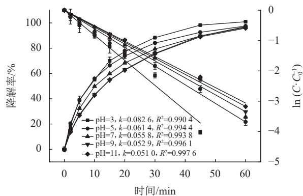
图 7 pH值对降解SAC的降解率影响
