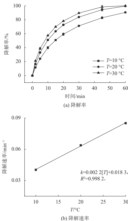
图8 水温对降解SAC的降解率和降解速率的影响
