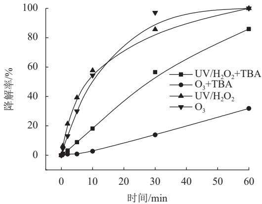
图 2 叔丁醇对UV/H 2 O 2 及臭氧氧化降解SAC的降解率的影响
