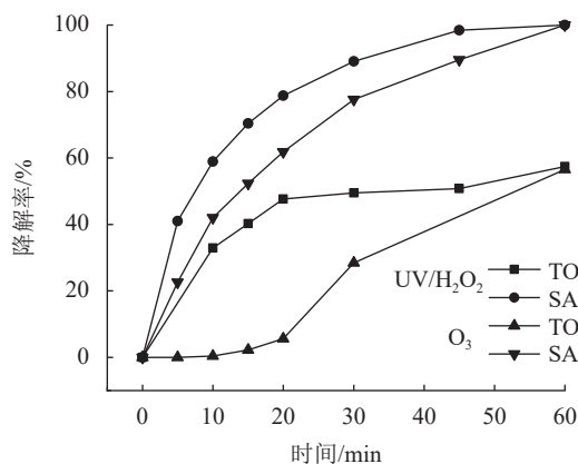
(b) 以 TOC 为指标的 SAC 降解效率
